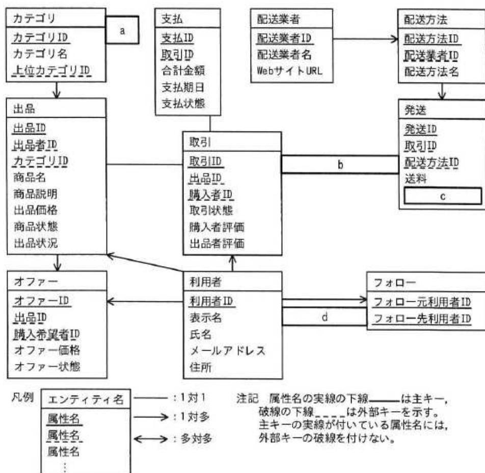
図 1 本システムの概念データモデル（抜粋）
